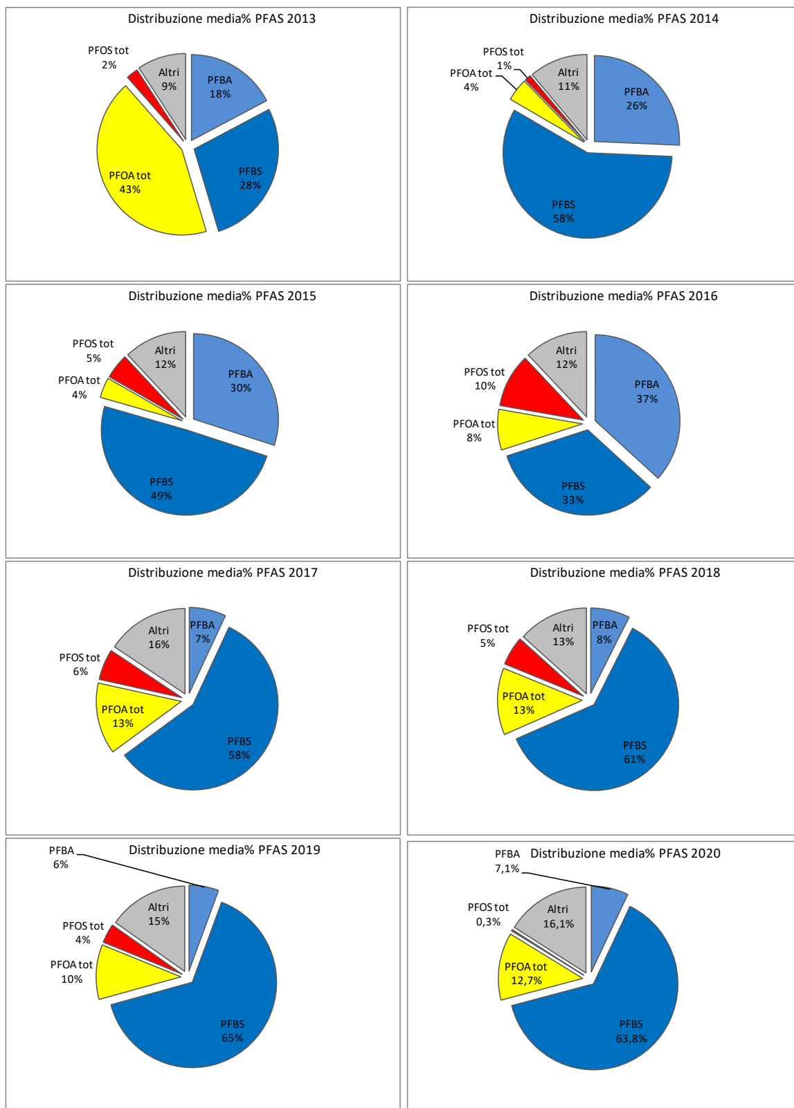
Figura 4-11 – Composizione percentuale delle diverse tipologie di PFAS dal 2013 al 2020
