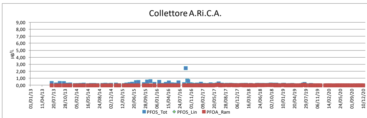
Figura 4-10 – Concentrazione di PFOS nel tempo per il collettore A.Ri.C.A. dal 2013 al 2020
