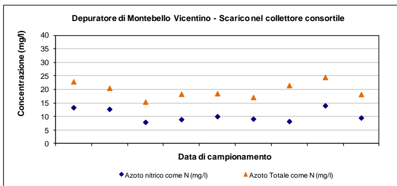
Figura 3-15 – Depuratore di Montebello Vic.: andamento di alcuni parametri allo scarico nel 2020
