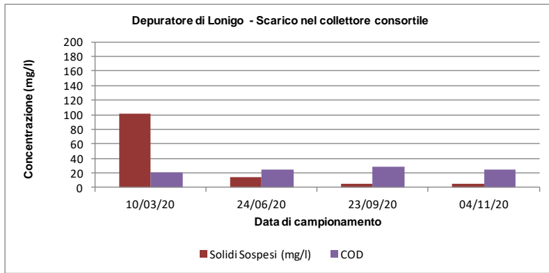
Figura 3-11 – Depuratore di Lonigo: andamento di COD e Solidi Sospesi per i Campioni in AIA 2020
