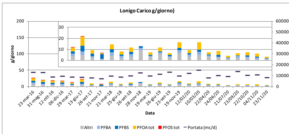
Figura 4-13 – Stima dei carichi PFAS (g/die) allo scarico del depuratore di Lonigo nel 2016-2020.
