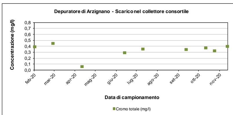
Figura 3-4 – Depuratore di Arzignano: andamento del cromo totale allo scarico nel 2020
