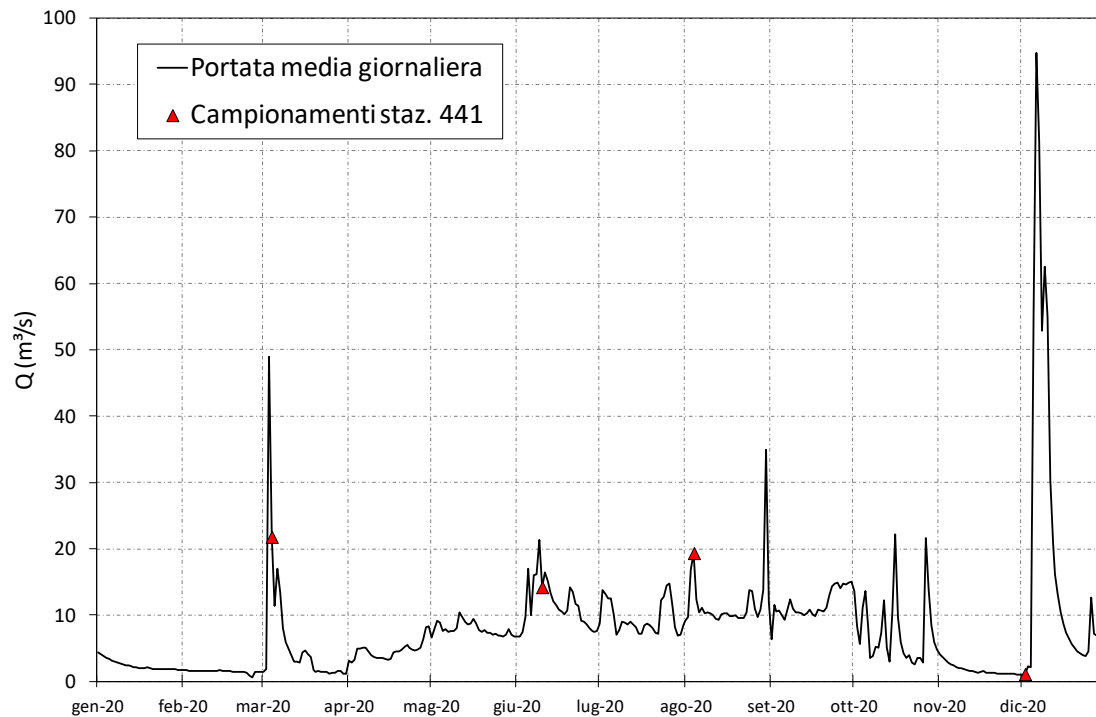
Figura 6-7 – Andamento delle portate medie giornaliere del fiume Frassine a Borgofrassine per l’anno 2020 con indicazione delle epoche di campionamento presso la stazione di Roveredo di Guà.
