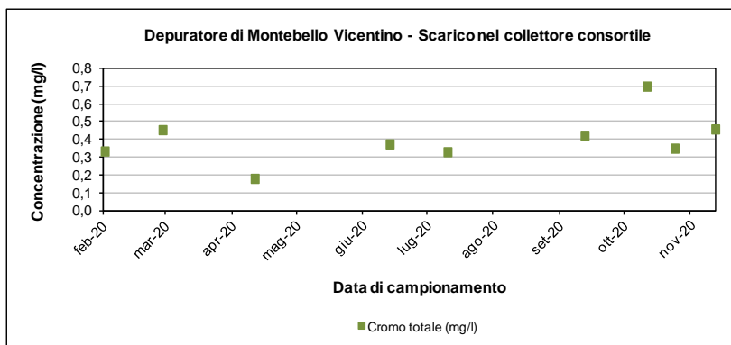
Figura 3-16 – Depuratore di Montebello Vic.: andamento del cromo totale allo scarico nel 2020
