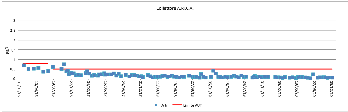
Figura 4-1 – Concentrazione di altri PFAS nel tempo per il collettore A.Ri.C.A. anno 2016-2020
