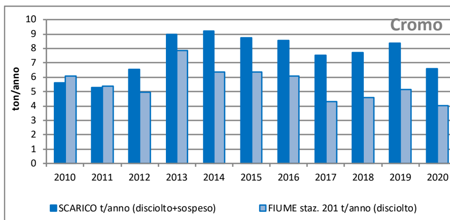
Figura 7-1 – Confronto tra i carichi di Cromo immessi dal collettore e quelli misurati molto più a valle nel Gorzone a Stanghella dal 2010 al 2020.
