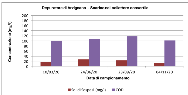
Figura 3-5 – Depuratore di Arzignano: andamento di COD e Solidi Sospesi per i Campioni in AIA 2020
