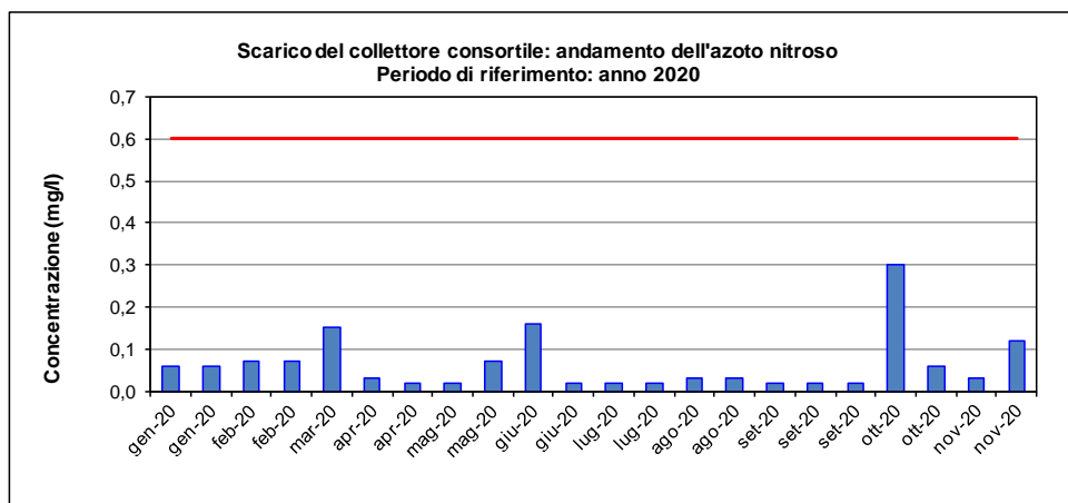
Figura 2-6 – Scarico del collettore consortile nel Fratta: andamento dell'azoto nitroso
