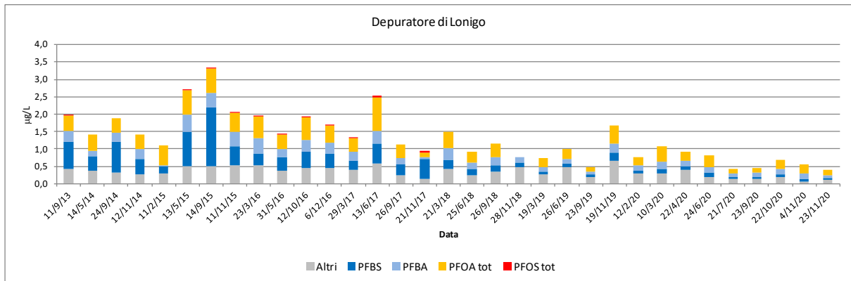
Figura 3-13- Depuratore di Lonigo: Composizione dei PFAS allo scarico 2013-2020
