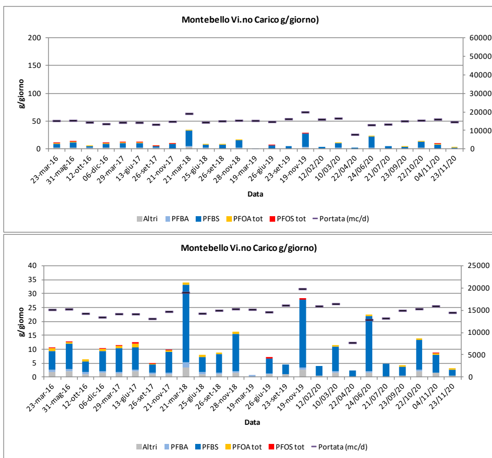
Figura 4-14 – Stima dei carichi PFAS (g/die) allo scarico del depuratore di Montebello Vicentino nel 2016-2020 con due scale diverse.
