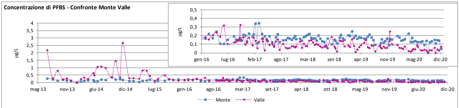
Figura 5-13 - Concentrazione di PFAS nelle stazioni poste 300 mt a monte del collettore A.Ri.C.A. e 200 mt a valle dello stesso dal 2013 al 2020
