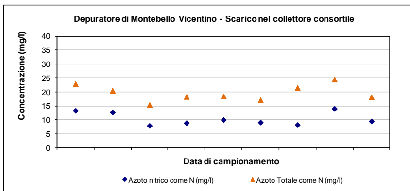
Figura 3-21 – Depuratore di Montecchio Magg.: andamento di alcuni parametri allo scarico nel 2020
