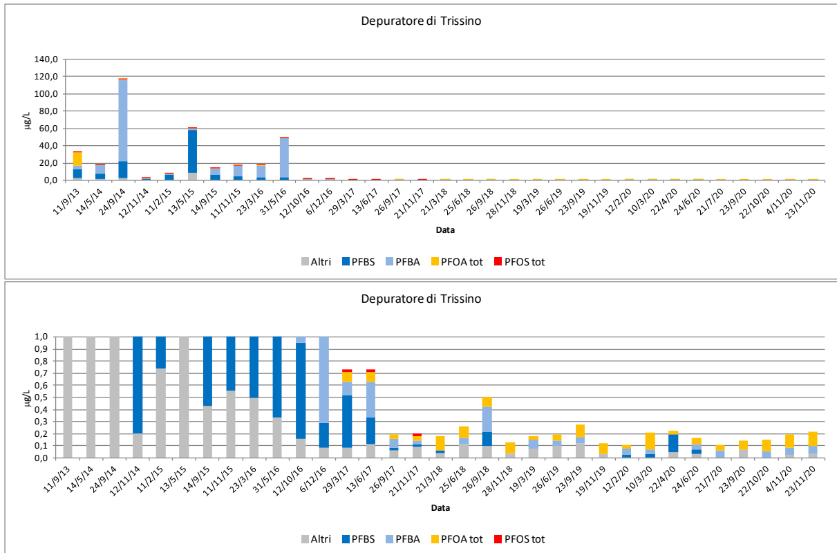
Figura 3-31 - Depuratore di Trissino: Composizione dei PFAS allo scarico 2013-2020 con sue scale diverse
