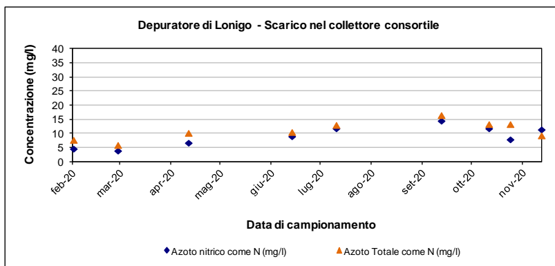
Figura 3-9 – Depuratore di Lonigo: andamento di alcuni parametri allo scarico nel 2020
