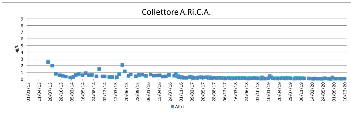
Figura 4-2 – Concentrazione di Altri PFAS nel tempo per il collettore A.Ri.C.A. dal 2013 al 2020
