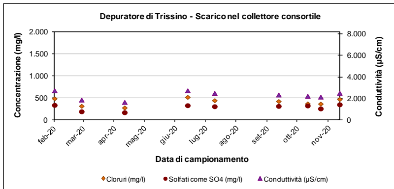
Figura 3-26 – Depuratore di Trissino: andamento di alcuni parametri allo scarico nel 2020
