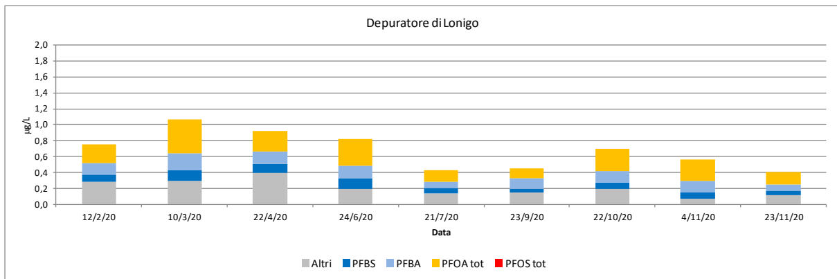
Figura 3-12 - Depuratore di Lonigo: Composizione dei PFAS allo scarico nel 2020
