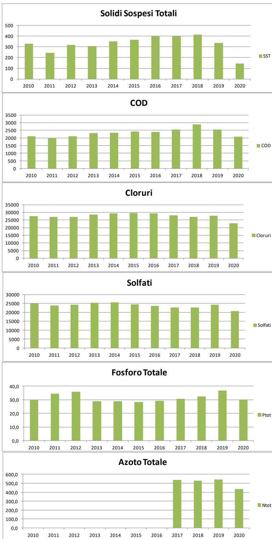
Figura 2-23 – Tendenza dei carichi espressi in tonnellate (riferimento a Tabella 1-2) nel periodo 2010 – 2020. L'azoto totale è stato determinato a partire dal 2017.
