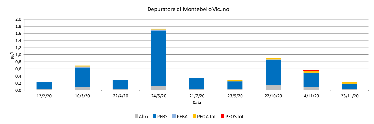
Figura 3-18 - Depuratore di Montebello Vic.no: Composizione dei PFAS allo scarico nel 2020
