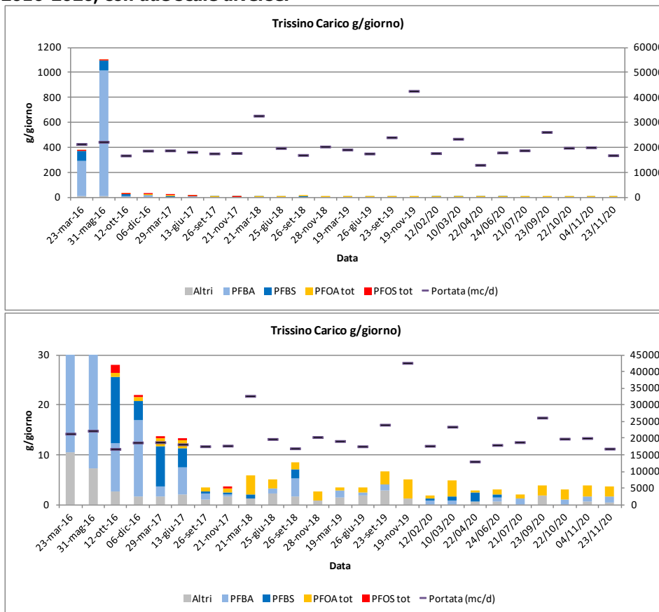
Figura 4-16 – Stima dei carichi PFAS (g/die) allo scarico del depuratore di Trissino nel 2016-2020, con due scale diverse.
