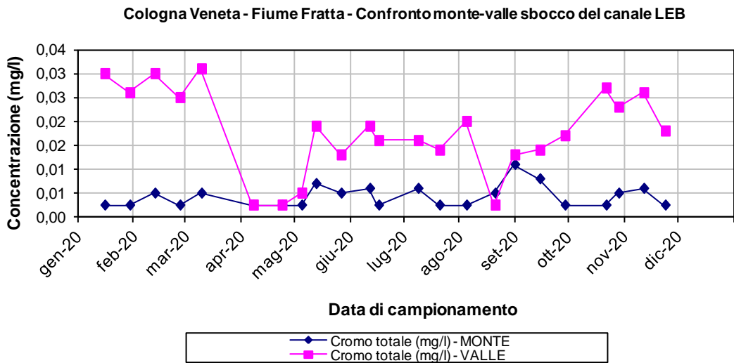
Figura 5-9 – Fiume Fratta: confronto monte/valle per il Cromo totale
