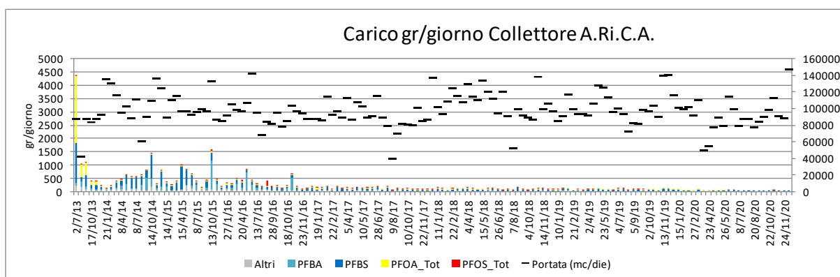
Figura 4-18 – Stima dei carichi PFAS (g/die) allo scarico del collettore A.Ri.C.A. dal 2013 al 2020.
