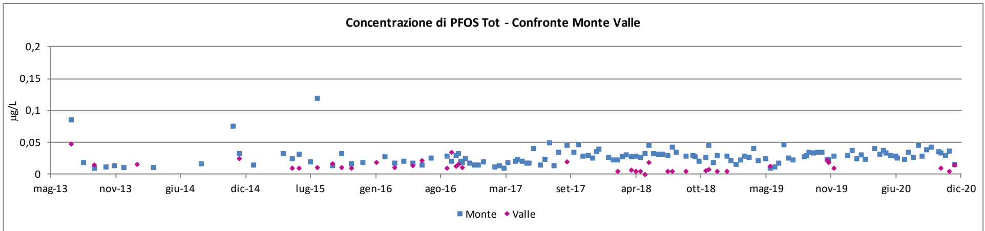
Figura 5-14 - Concentrazione di PFAS nelle stazioni poste 300 mt a monte del collettore A.Ri.C.A. e 200 mt a valle dello stesso dal 2013 al 2020
