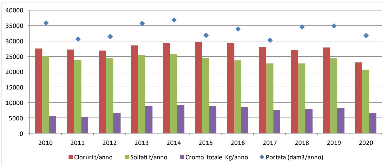
Figura 2-22 – Tendenza dei carichi espressi in tonnellate per Cloruri e Solfati ed in chilogrammi per il Cromo nel periodo 2010 – 2020.
