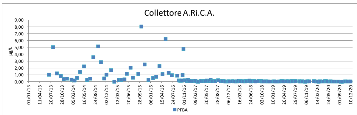
Figura 4-4 – Concentrazione di PFBA nel tempo per il collettore A.Ri.C.A. dal 2013 al 2020
