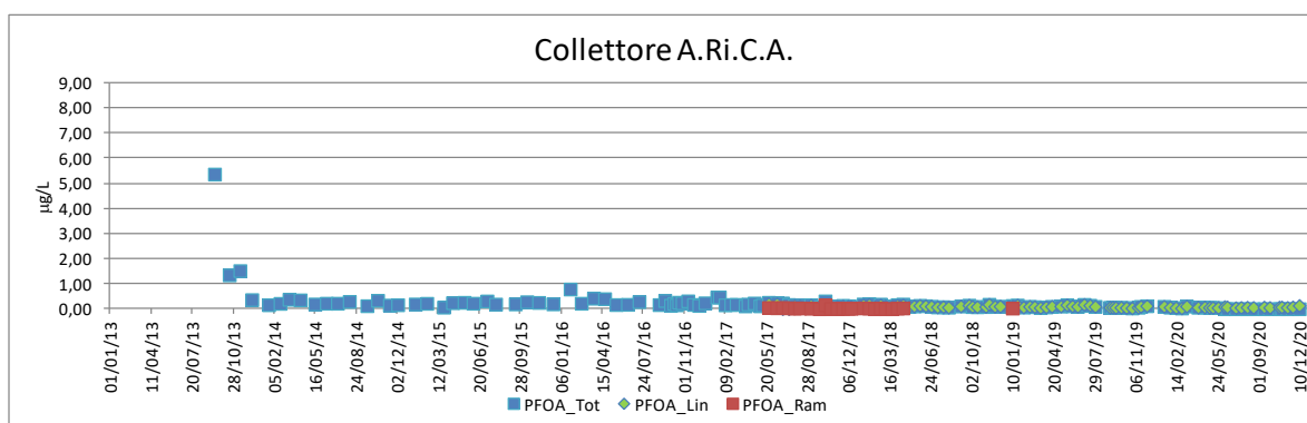
Figura 4-8 – Concentrazione di PFOA nel tempo per il collettore A.Ri.C.A. dal 2013 al 2020
