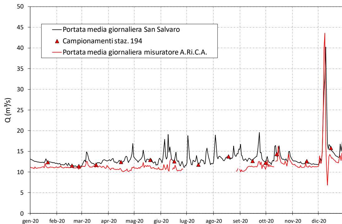
Figura 6-6 – Portate medie giornaliere del fiume Fratta a San Salvaro e portate medie giornaliere del fiume Fratta a Cologna Veneta fornite da A.Ri.C.A. per l’anno 2020.
