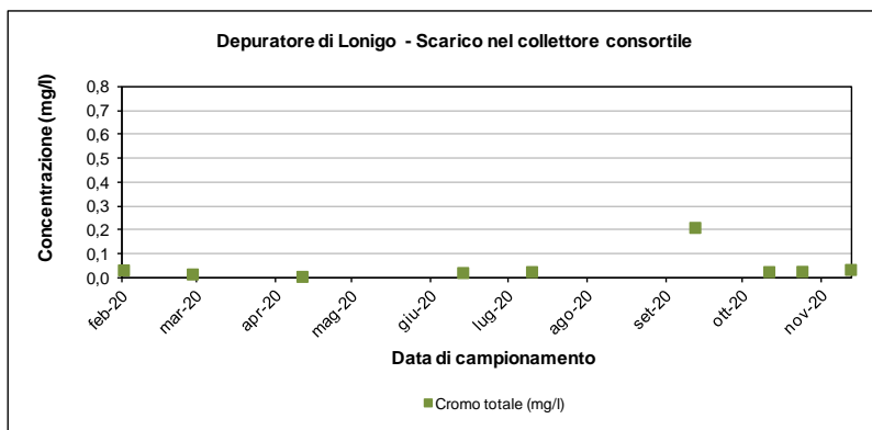
Figura 3-10 – Depuratore di Lonigo: andamento del cromo totale allo scarico nel 2020
