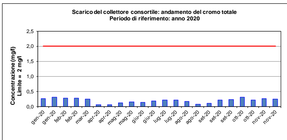
Figura 2-9 – Scarico del collettore consortile nel Fratta: andamento del cromo totale
