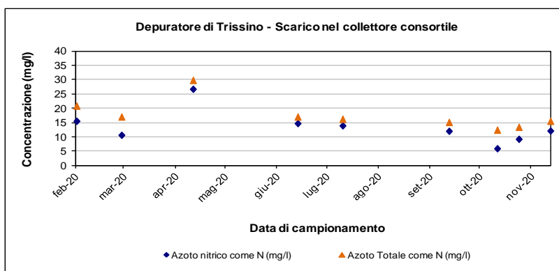
Figura 3-27 – Depuratore di Trissino: andamento di alcuni parametri allo scarico nel 2020
