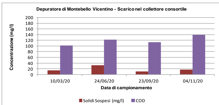
Figura 3-23 – Depuratore di Montecchio Magg: andamento di COD e Solidi Sospesi per i Campioni in AIA 2020
