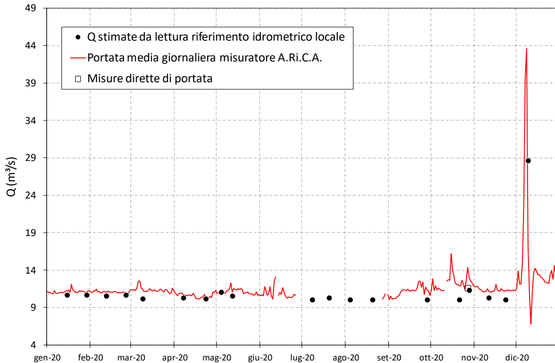
Figura 6-8. Portate medie giornaliere (dati A.Ri.C.A.) del fiume Fratta a valle del rilascio del canale L.E.B. con indicazione delle misure eseguite da ARPAV e dei valori di portata ricavati da scala di deflusso sulla base delle letture operate nei giorni di campionamento qualitativo presso la stazione 2105.
