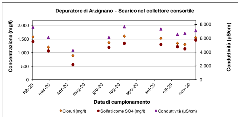
Figura 3-2 – Depuratore di Arzignano: andamento di alcuni parametri allo scarico nel 2020
