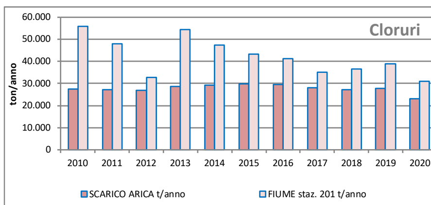
Figura 7-2 – Confronto tra i carichi di Cloruri immessi dal collettore e quelli misurati molto più a valle nel Gorzone a Stanghella dal 2010 al 2020.
