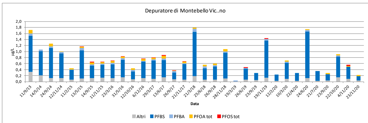
Figura 3-19- Depuratore di Montebello Vic.no: Composizione dei PFAS allo scarico 2013-2020
