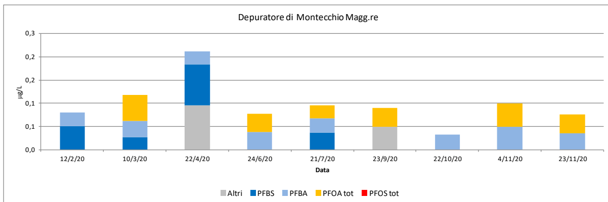
Figura 3-24 - Depuratore di Montecchio Magg.re: Composizione dei PFAS allo scarico nel 2020 con due scale diverse
