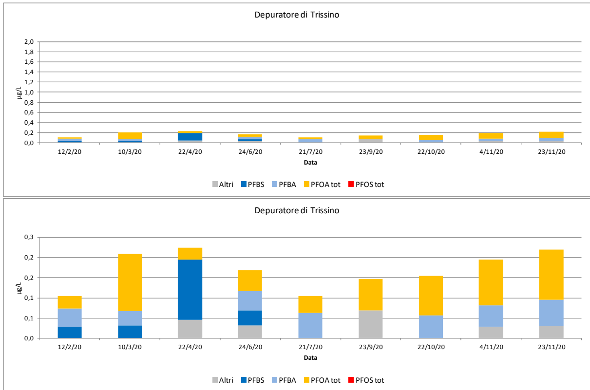
Figura 3-30 - Depuratore di Trissino: Composizione dei PFAS allo scarico nel 2020 con sue scale diverse
