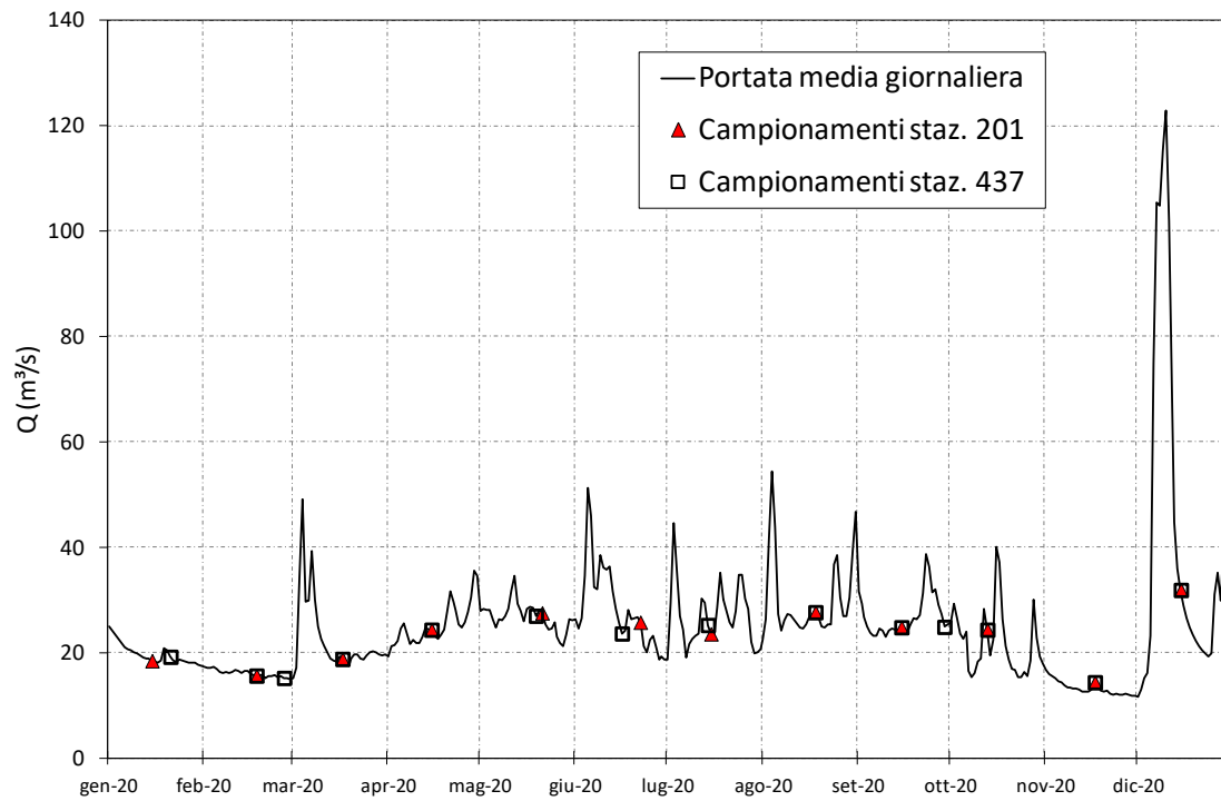
Figura 6-5 – Portate del Fiume Gorzone a Stanghella nell’anno 2020, con indicazione delle epoche dei campionamenti di qualità a Stanghella (201) e a Valcerere Dolfina (437).
