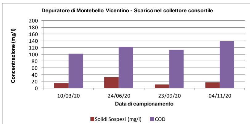
Figura 3-17 – Depuratore di Montebello Vic: andamento di COD e Solidi Sospesi per i Campioni in AIA 2020.
