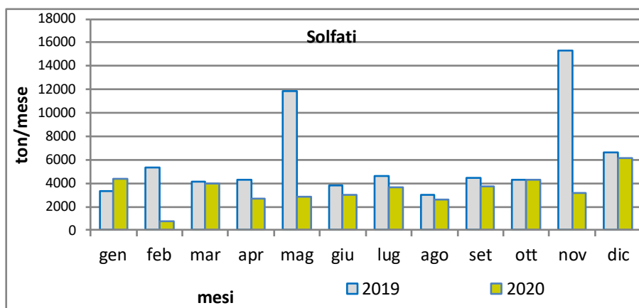
Figura 7-5 – Stima del carico medio mensile di Cloruri nel Fiume Gorzone a Stanghella nell'anno 2020 e confronto con l'anno precedente.
