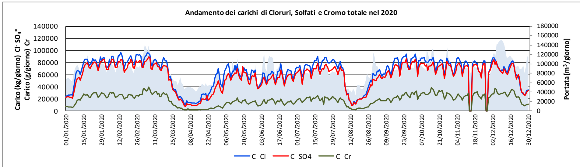
Figura 2-21 – Andamento dei carichi
