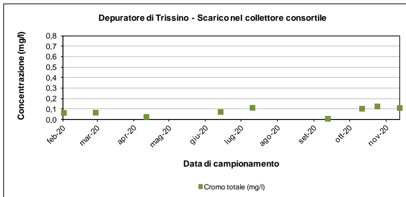
Figura 3-28 – Depuratore di Trissino: andamento del cromo totale allo scarico nel 2020
