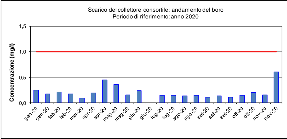
Figura 2-11 – Scarico del collettore consortile nel Fratta: andamento del boro
