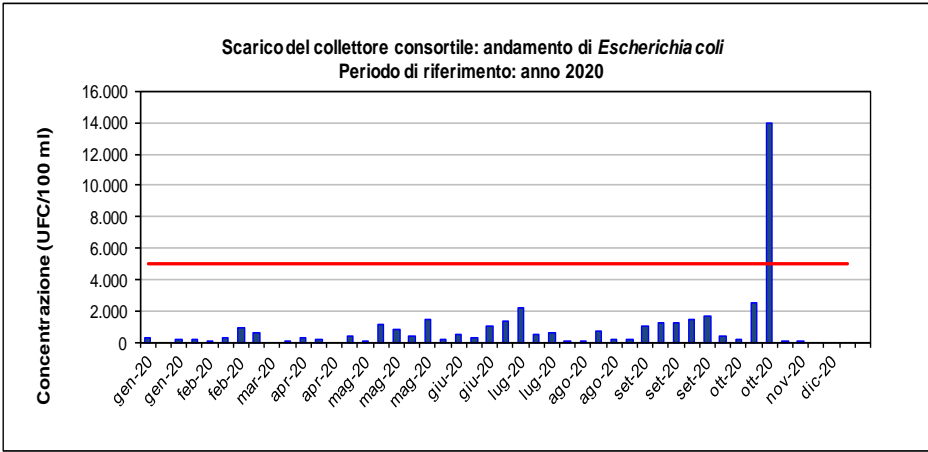
Figura 2-10 – Scarico del collettore consortile nel Fratta: andamento degli Escherichia coli
