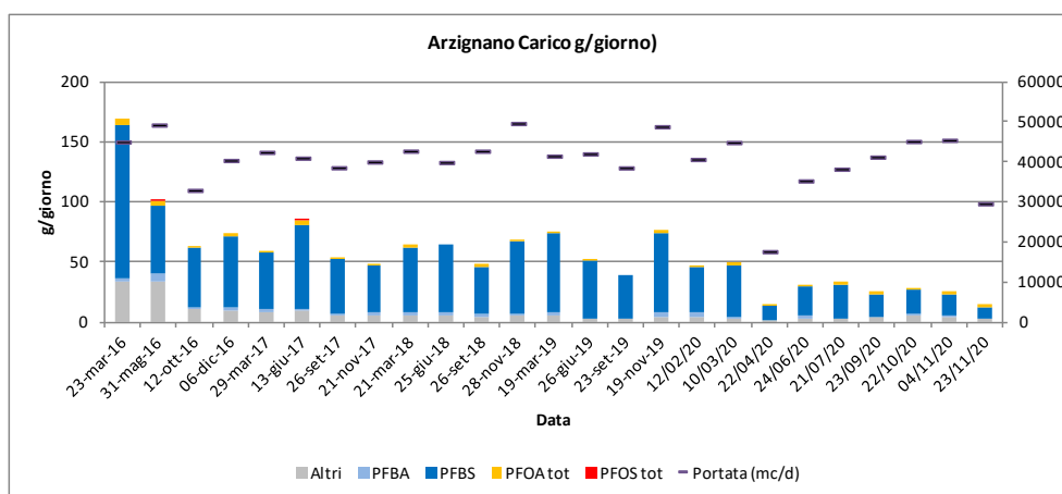
Figura 4-12 – Stima dei carichi PFAS (g/die) allo scarico del depuratore di Arzignano nel 2016-2020.
