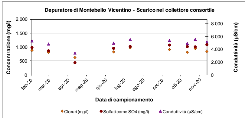
Figura 3-14 – Depuratore di Montebello Vic.: andamento di alcuni parametri allo scarico nel 2020
