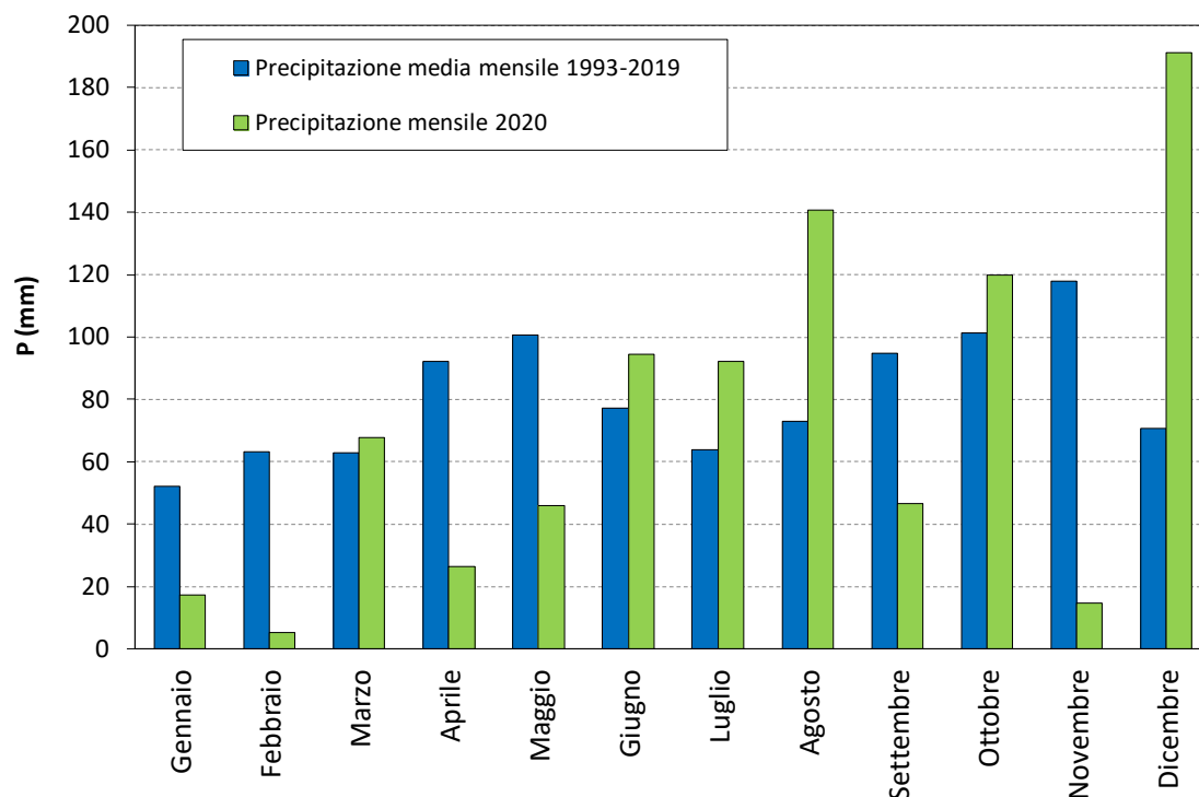
Figura 6-1 – Confronto tra i valori spazializzati a scala di bacino (Fratta-Gorzone chiuso a Stanghella) delle precipitazioni medie mensili del periodo 1993-2019 e cumulate mensili del 2020.
