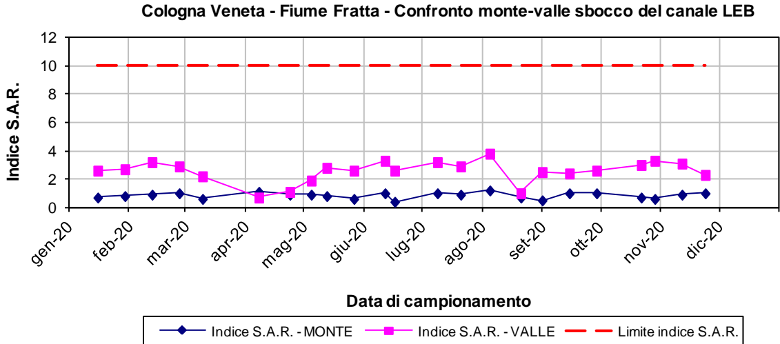
Figura 5-8 – Fiume Fratta: confronto monte/valle per l'Indice S.A.R.
