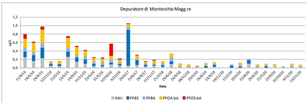
Figura 3-25 - Depuratore di Montecchio Magg.re: Composizione dei PFAS allo scarico 2013-2020 con due scale diverse
