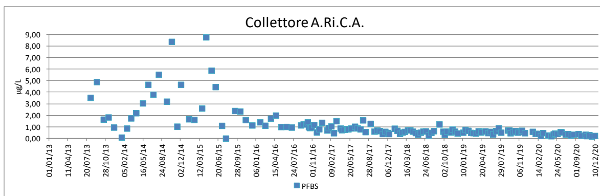
Figura 4-6 – Concentrazione di PFBS nel tempo per il collettore A.Ri.C.A. dal 2013 al 2020
