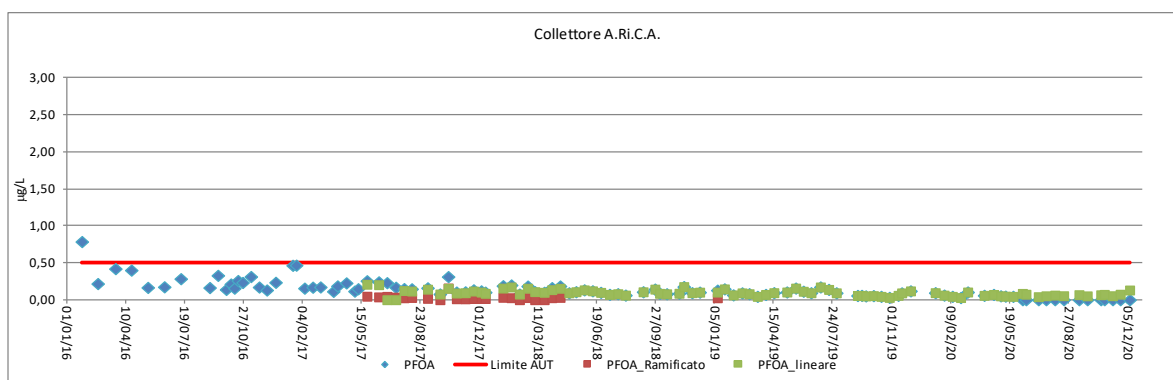
Figura 4-7 – Concentrazione di PFOA nel tempo per il collettore A.Ri.C.A. anno 2016-2020
