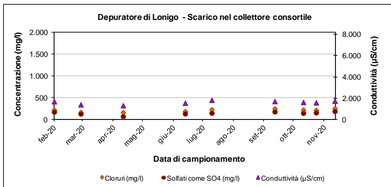
Figura 3-8 – Depuratore di Lonigo: andamento di alcuni parametri allo scarico nel 2020
