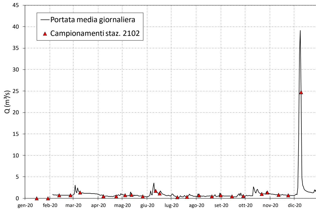
Figura 6-9 – Portate medie giornaliere del fiume Tegna a Cologna Veneta presso la stazione di monitoraggio qualitativo numero 2102.
