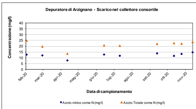
Figura 3-3 – Depuratore di Arzignano: andamento di alcuni parametri allo scarico nel 2020
