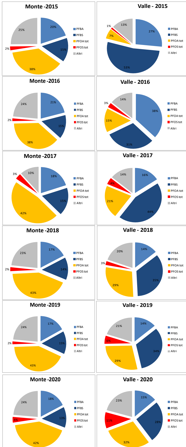
Figura 5-18 - Composizione percentuale dei carichi medi giornalieri a monte e a valle del collettore A.Ri.C.A. dal 2015 al 2020
