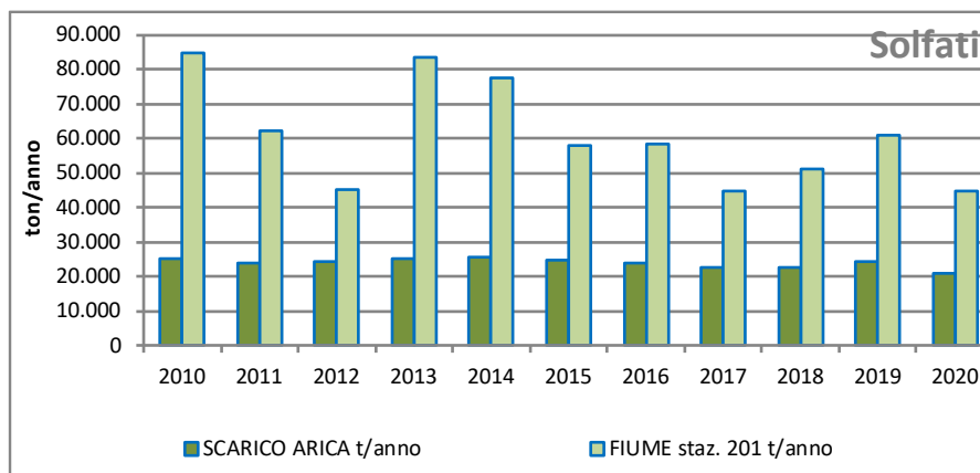
Figura 7-3 – Confronto tra i carichi di Solfati immessi dal collettore e quelli misurati molto più a valle nel Gorzone a Stanghella dal 2010 al 2020.
