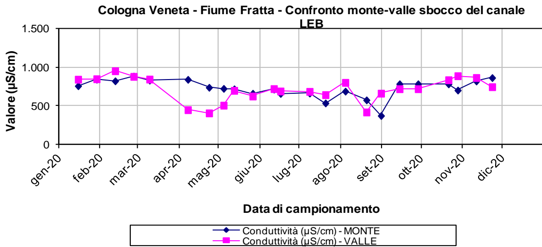
Figura 5-6 – Fiume Fratta: confronto monte/valle per la Conduttività
