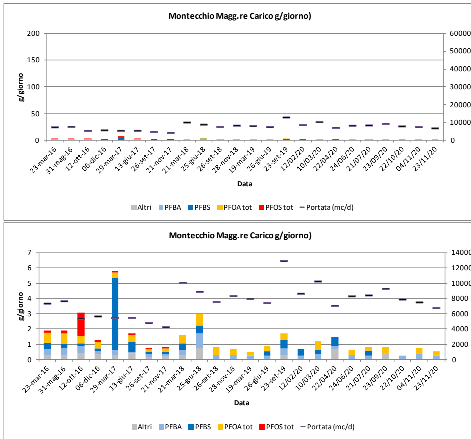
Figura 4-15 – Stima dei carichi PFAS (g/die) allo scarico del depuratore di Montecchio Maggiore nel 2016-2020, con due scale diverse.
