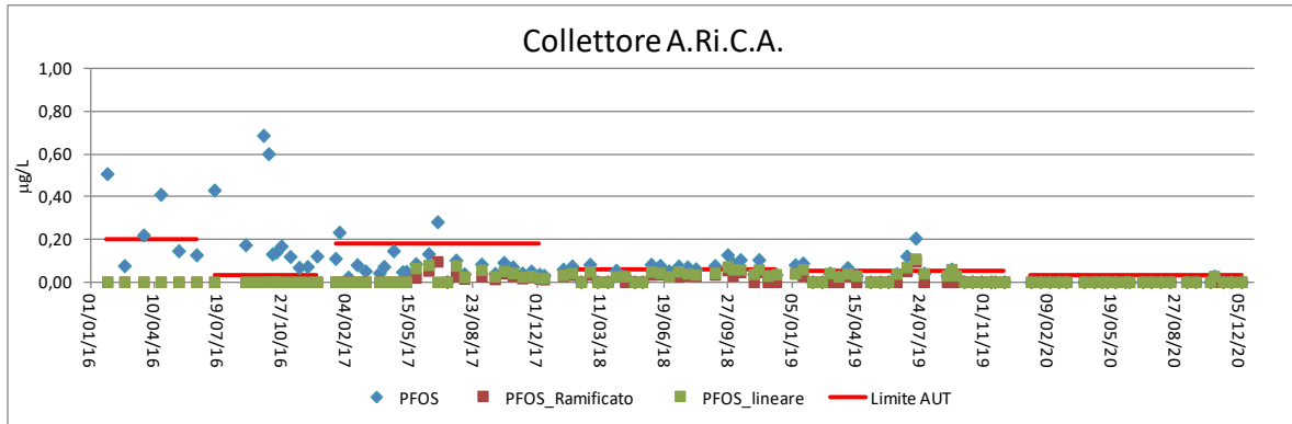
Figura 4-9 – Concentrazione di PFOS nel tempo per il collettore A.Ri.C.A. anno 2016-2020
