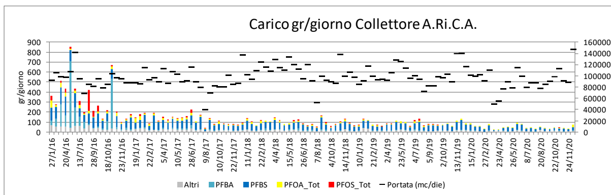
Figura 4-17 – Stima dei carichi PFAS (g/die) allo scarico del collettore A.Ri.C.A. nel 2016-2020. La scala è maggiore rispetto a quella dei singoli depuratori per avere una visione completa dei singoli contributi.
