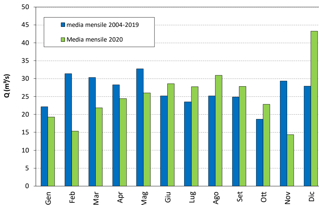
Figura 6-10 – Confronto tra l'andamento delle portate medie mensili del 2020 e delle portate medie mensili della serie storica di osservazioni disponibile (2004-2019) per la sezione di Stanghella.
