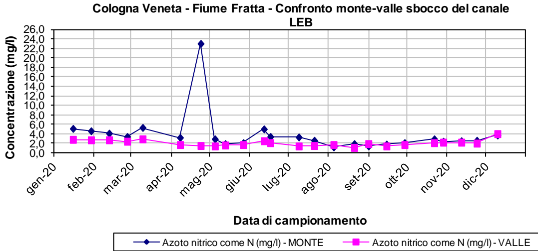
Figura 5-2 – Fiume Fratta: confronto monte/valle per l’Azoto nitrico (l’ultimo dato di valle è senza la diluizione del L.E.B.)
