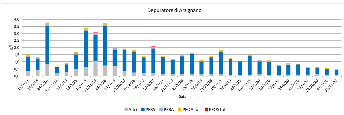
Figura 3-6 - Depuratore di Arzignano: Composizione dei PFAS allo scarico nel 2020
