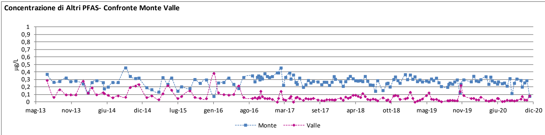
Figura 5-16 - Concentrazione di PFAS nelle stazioni poste 300 mt a monte del collettore A.Ri.C.A. e 200 mt a valle dello stesso dal 2013 al 2020
