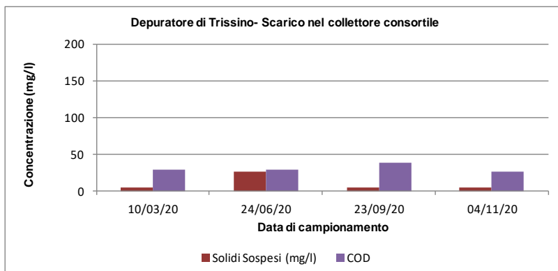
Figura 3-29 – Depuratore di Trissino: andamento di COD e Solidi Sospesi per i Campioni in AIA 2020
