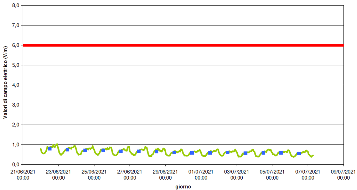
Misure di campo elettrico (V/m) Scuola Isola del Tesoro Dolo
