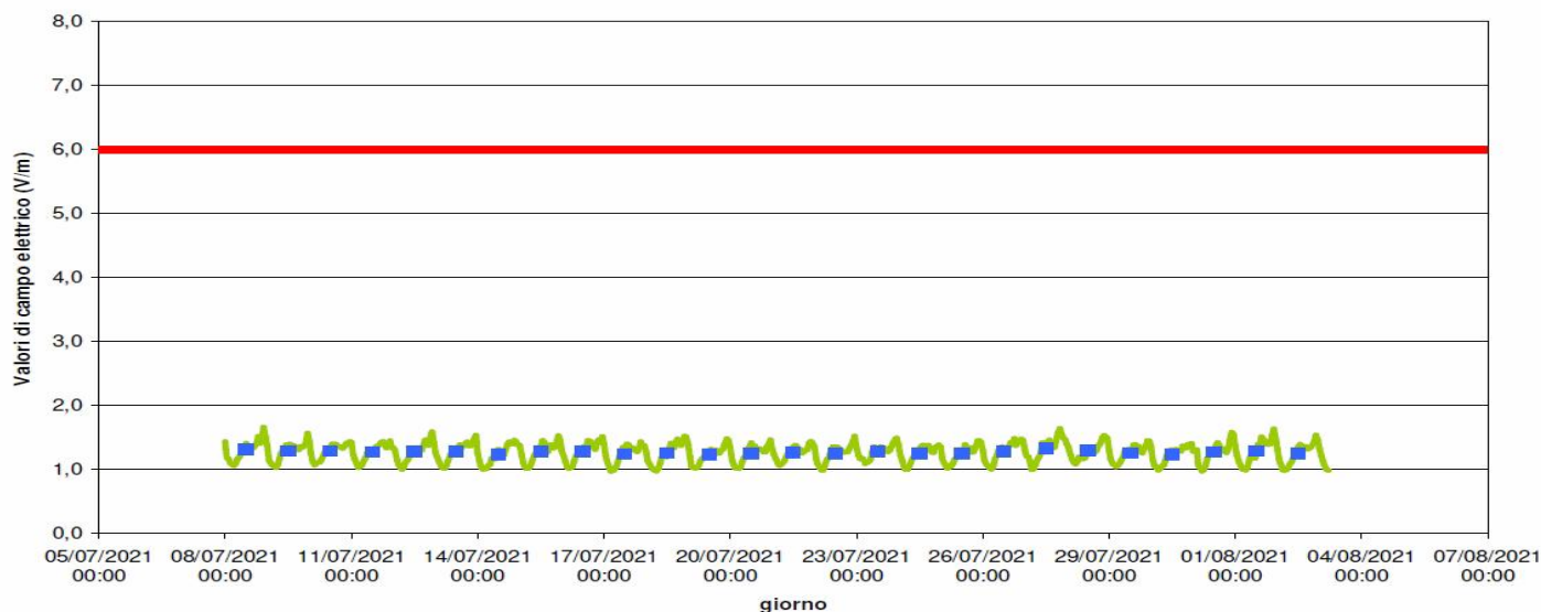
Misure di campo elettrico (V/m) Scuola Giotto Dolo
