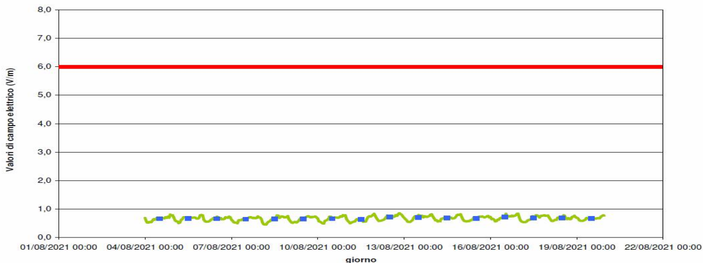
Misure di campo elettrico (V/m) Scuola De Amicis Dolo
