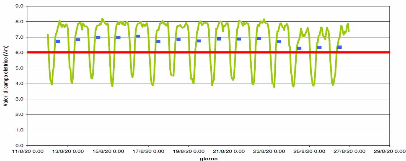
Misure di campo elettrico (V/m) via Dante Alighieri, 44A Jesolo
