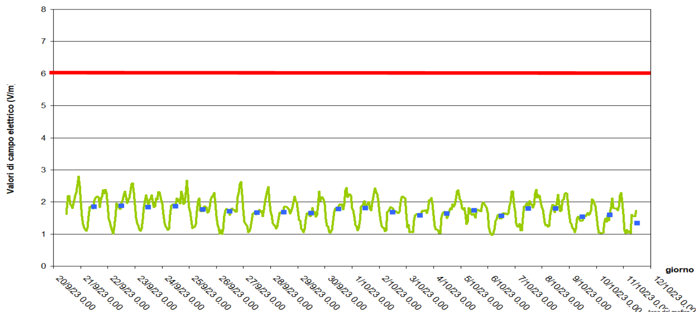
Misure di campo elettrico (V/m) via della Vega 11, Bibione - San Michele al Tagliamento
