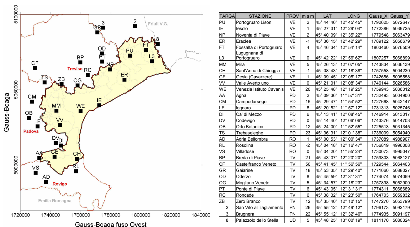
Figura 4.1: Ubicazione ed elenco delle stazioni meteorologiche del Centro Meteorologico di Teolo e dell'Osservatorio Meteorologico della Regione Friuli Venezia-Giulia, utilizzate per l'analisi del periodo 1992-2004.
