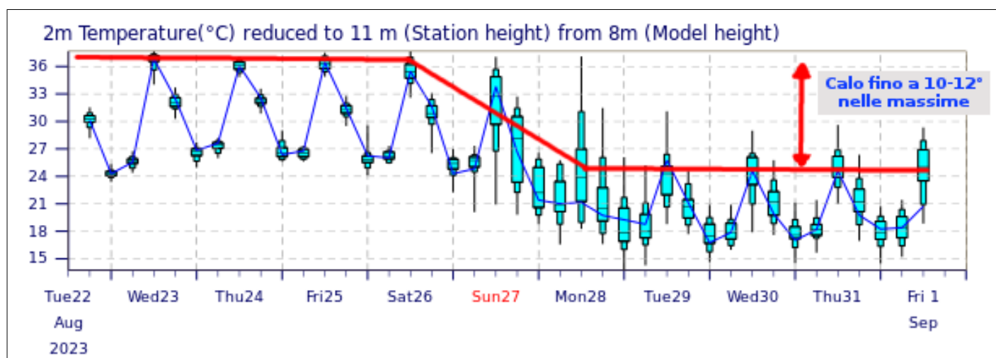
Figura 2 - Previsione probabilistica (Modello Ensemble di ECMWF) dell'andamento di temperatura a 2 metri nella città di Padova; si osserva il calo marcato delle temperature previsto tra domenica 27 e lunedì 28 agosto
