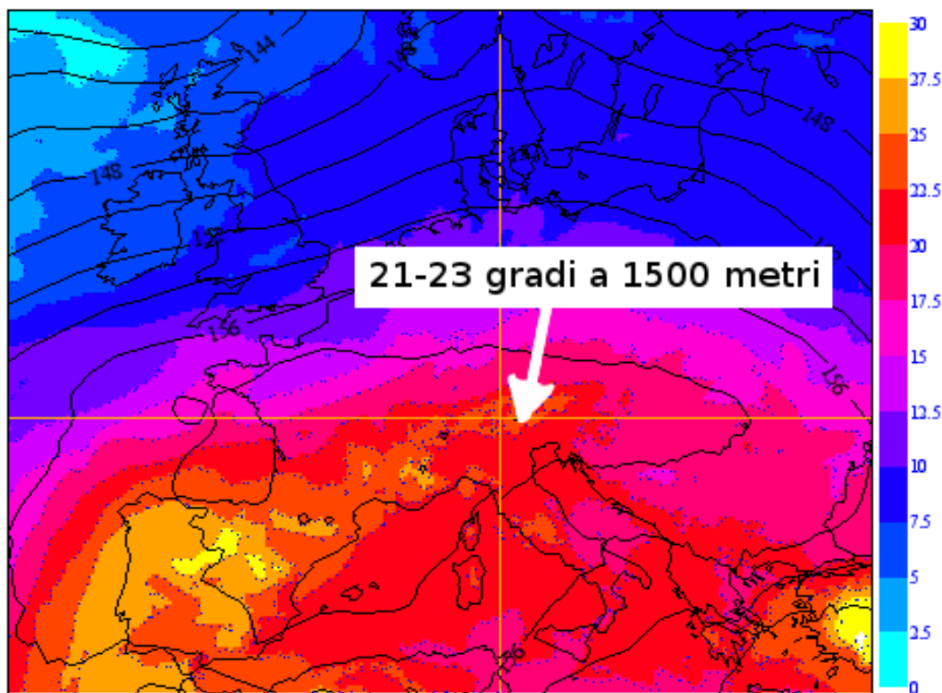
Figura 1 - Situazione prevista per mercoledì 23 agosto alle ore 12.00, temperatura a 850 mbar (1500-1600 metri di quota). Si osserva la massa di aria calda estesa dal sudovest d'Europa fino all'Italia settentrionale, con temperature molto alte associate all'anticiclone. (Mappa ricavata dai dati del Modello meteorologico di ECMWF)
