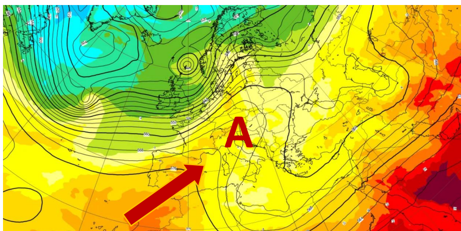
immagine del modello ECMWF (run 00 del 30/03/2026)
