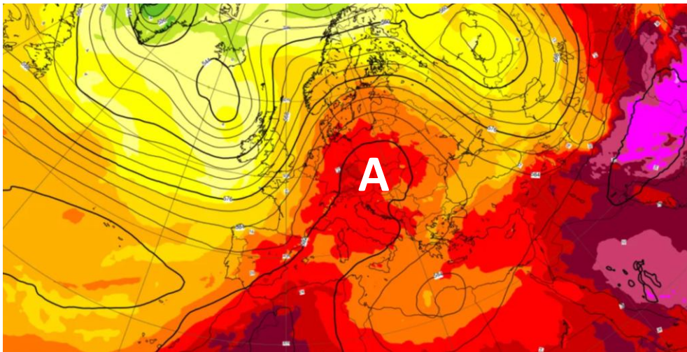
Fig.2-Mappa del geopotenziale a 500hPa-temperature 850hPa del modello globale ECMWF, prevista per domenica 28 giugno (ore 12 UTC), dove si può notare la vasta area di alta pressione associata ad aria calda di origine sub-tropicale
