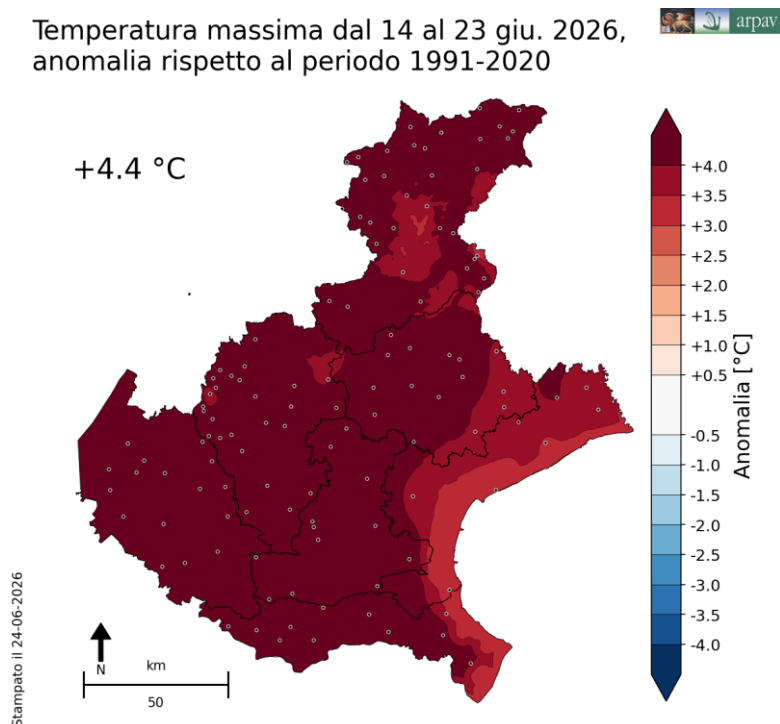
Fig.1- anomalia di temperatura massima registrata nel periodo 14-23 giugno 2026 confrontata con i dati del periodo 1991-2020. Per ritrovare nella serie storica uno stesso periodo altrettanto caldo bisogna risalire a giugno 2002
