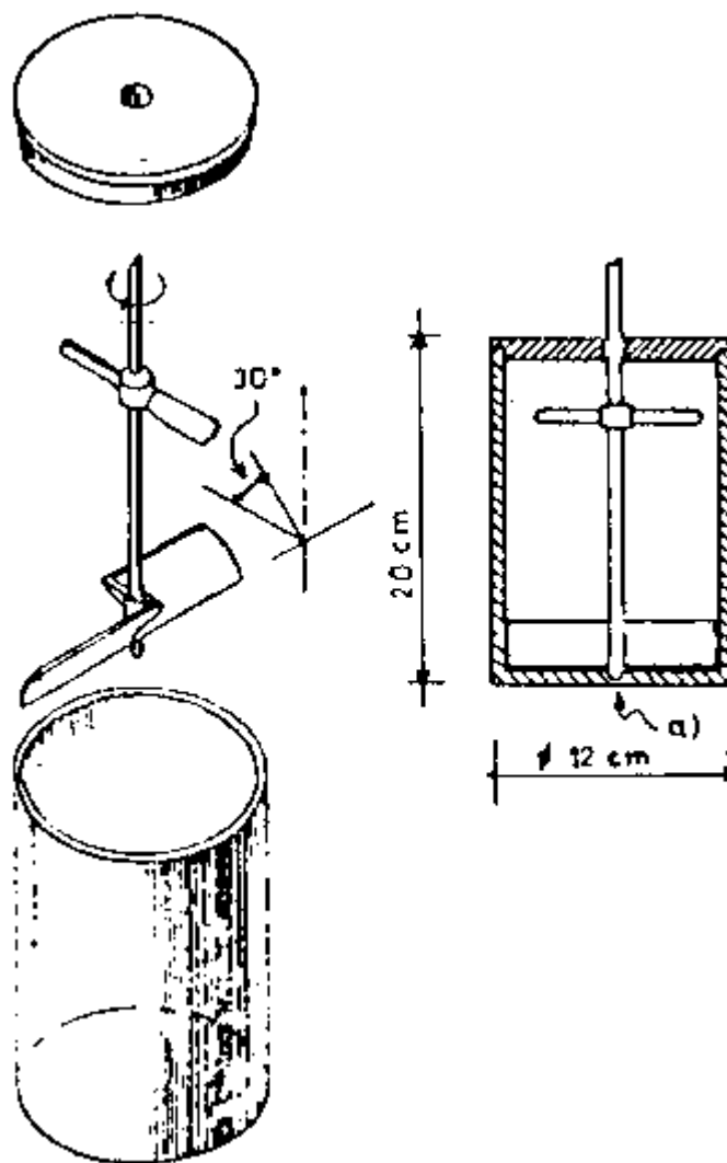
Figura 1 - Estrattore
