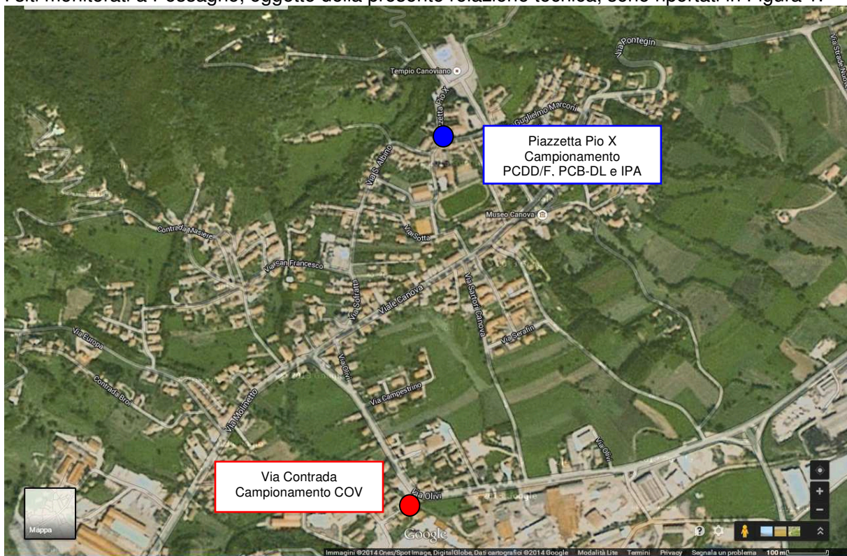
Figura 1- Comune di Possagno, siti monitorati per la determinazione di PCDD/F, PCB-DL, IPA e COV
