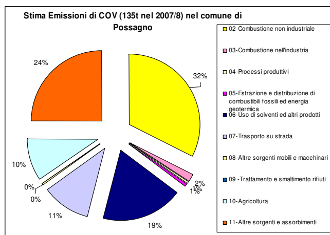
Figura 13 Contributi percentuali dei macrosettori CORINAIR alla stima emissioni di COV nel comune di Possagno – dati INEMAR 2007/8
