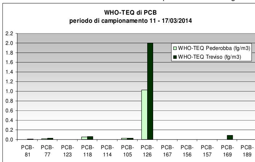
Figura 17 – Concentrazioni medie di PCB espresse come WHO -TEQ rilevati presso i siti di Possagno e Treviso
