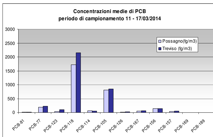
Figura 16 – Concentrazioni medie di PCB-DL rilevati presso i siti di Possagno e Treviso
