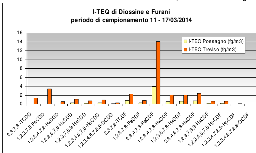
Figura 15 – Concentrazioni medie di diossine e furani espresse come I-TEQ rilevati presso i siti di Possagno e Treviso
