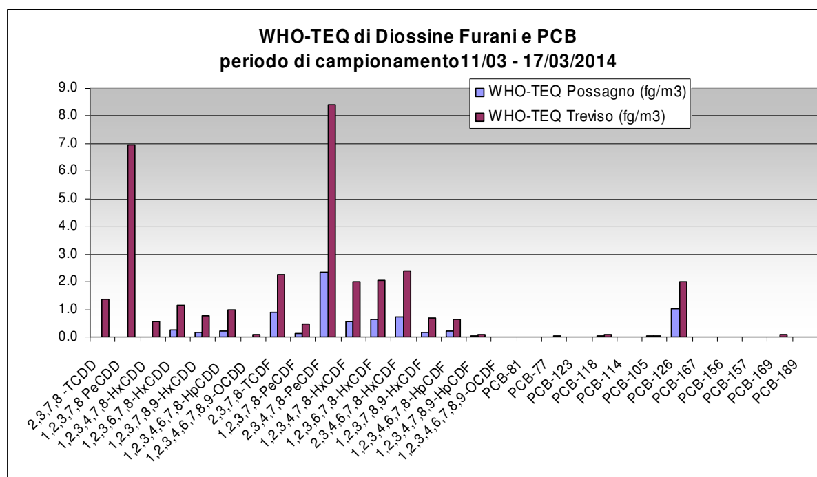
Figura 18 – Concentrazioni medie di Diossine, Furani e PCB espresse come WHO -TEQ rilevati presso i siti di Possagno e Treviso
