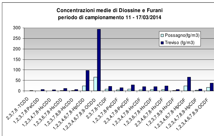
Figura 14 – Concentrazioni medie di diossine e furani rilevati presso i siti di Possagno e Treviso
