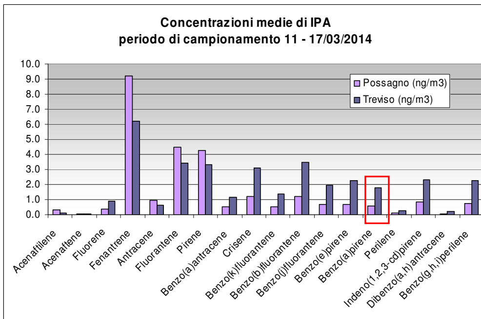
Figura 19 – Concentrazioni medie di IPA rilevati presso i siti di Possagno e Treviso
