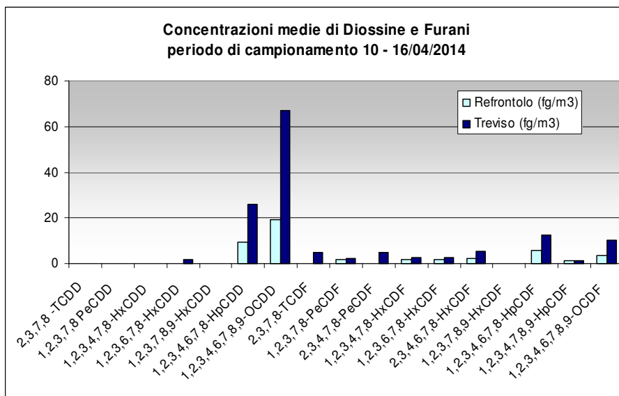
Figura 14 – Concentrazioni medie di diossine e furani rilevati presso i siti di Refrontolo e Treviso
