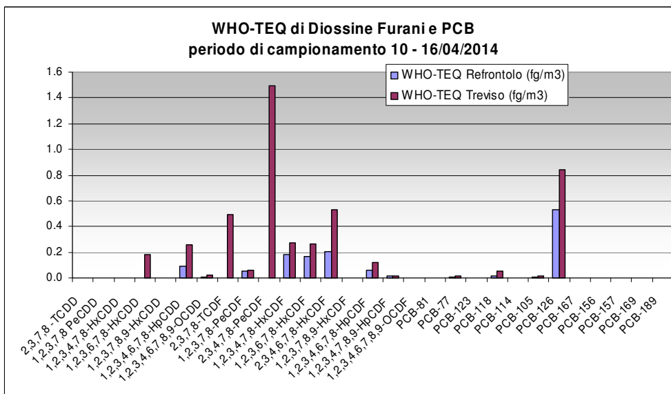
Figura 18 – Concentrazioni medie di Diossine, Furani e PCB espresse come WHO -TEQ rilevati presso i siti di Refrontolo e Treviso
