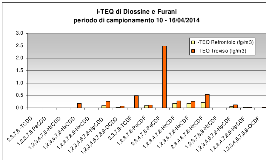
Figura 15 – Concentrazioni medie di diossine e furani espresse come I-TEQ rilevati presso i siti di Refrontolo e Treviso
