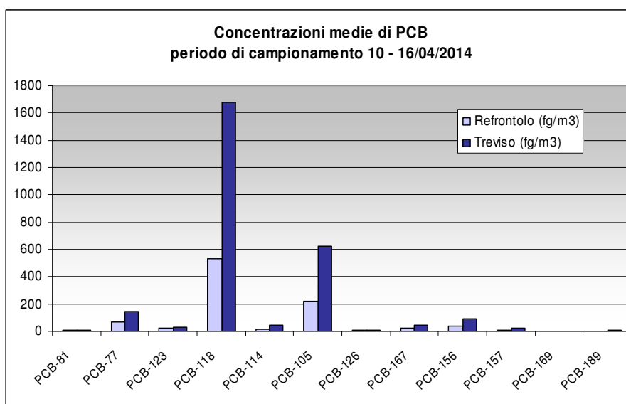
Figura 16 – Concentrazioni medie di PCB-DL rilevati presso i siti di Refrontolo e Treviso
