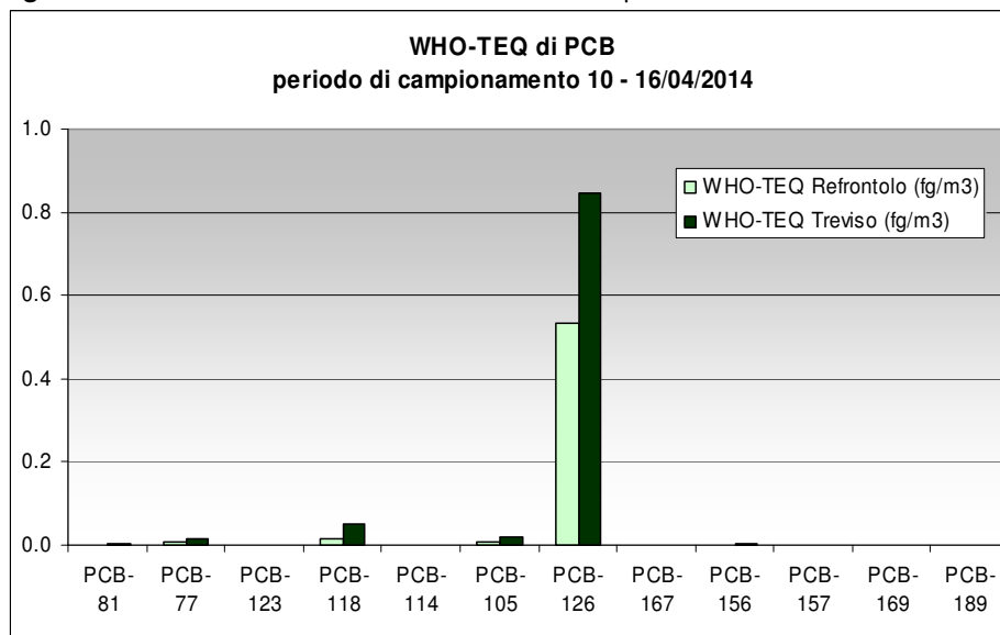
Figura 17 – Concentrazioni medie di PCB espresse come WHO -TEQ rilevati presso i siti di Refrontolo e Treviso
