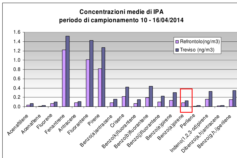
Figura 19 – Concentrazioni medie di IPA rilevati presso i siti di Refrontolo e Treviso
