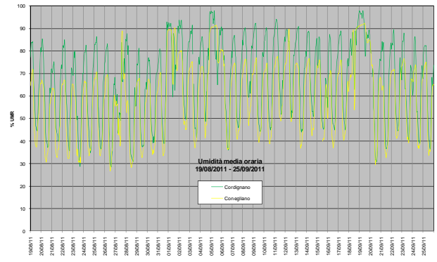
Grafico 20: Valori orari di umidità osservati presso la stazione rilocabile posizionata a Cordignano – campagna estiva
