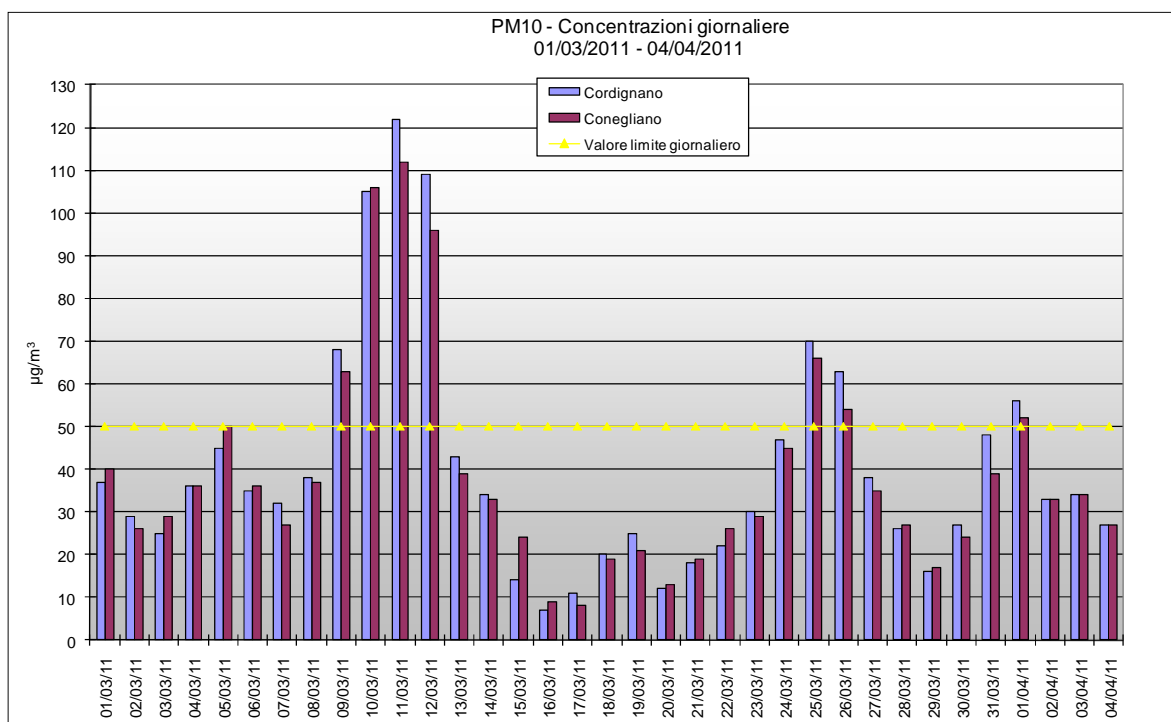
Grafico 10: Valori medi giornalieri di PM10 rilevati presso la stazione fissa di Conegliano e la stazione rilocabile posizionata a Cordignano – campagna invernale.
