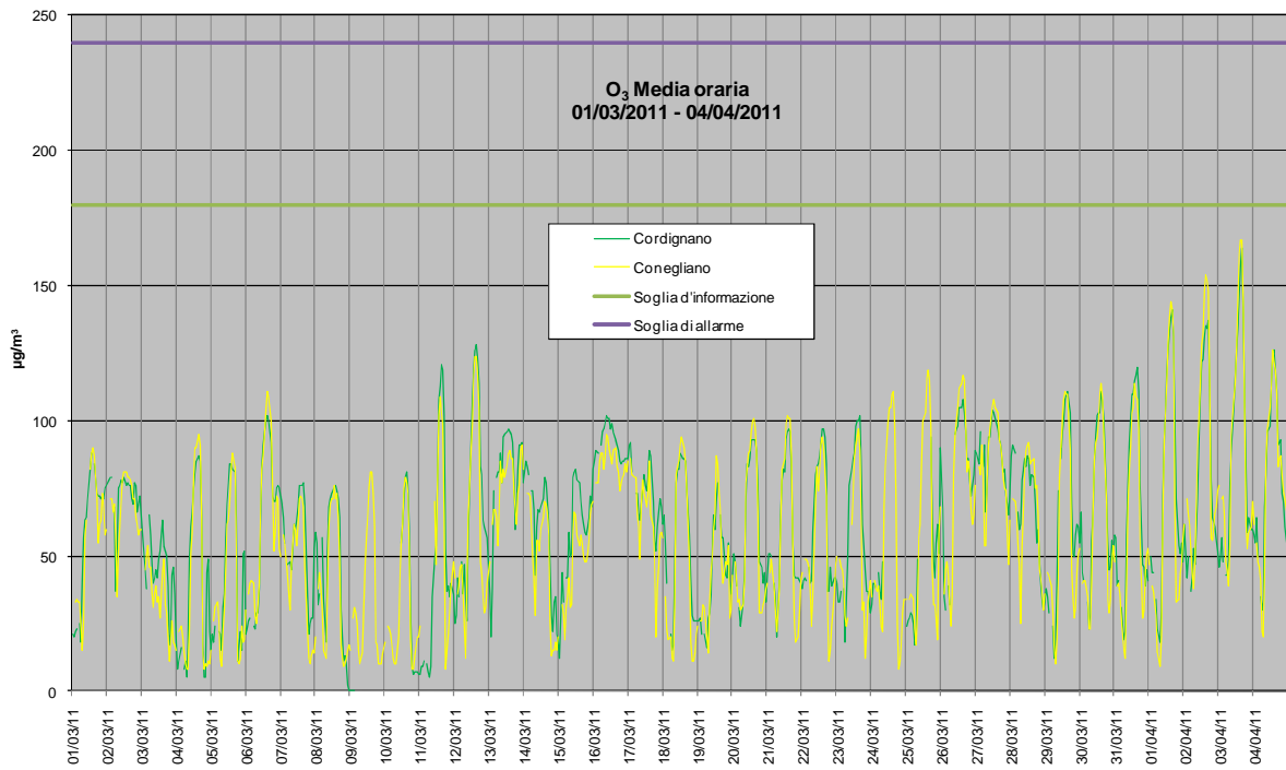
Grafico 5: Valori orari di O 3 rilevati presso la stazione fissa di Conegliano e la stazione rilocabile posizionata a Cordignano – campagna invernale.
