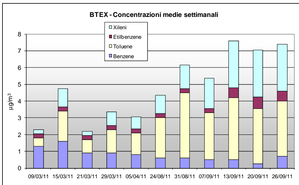
Grafico 12 Valori settimanali di BTEX (Benzene, Toluene, Etilbenzene, Xilene) rilevati a Cordignano.
