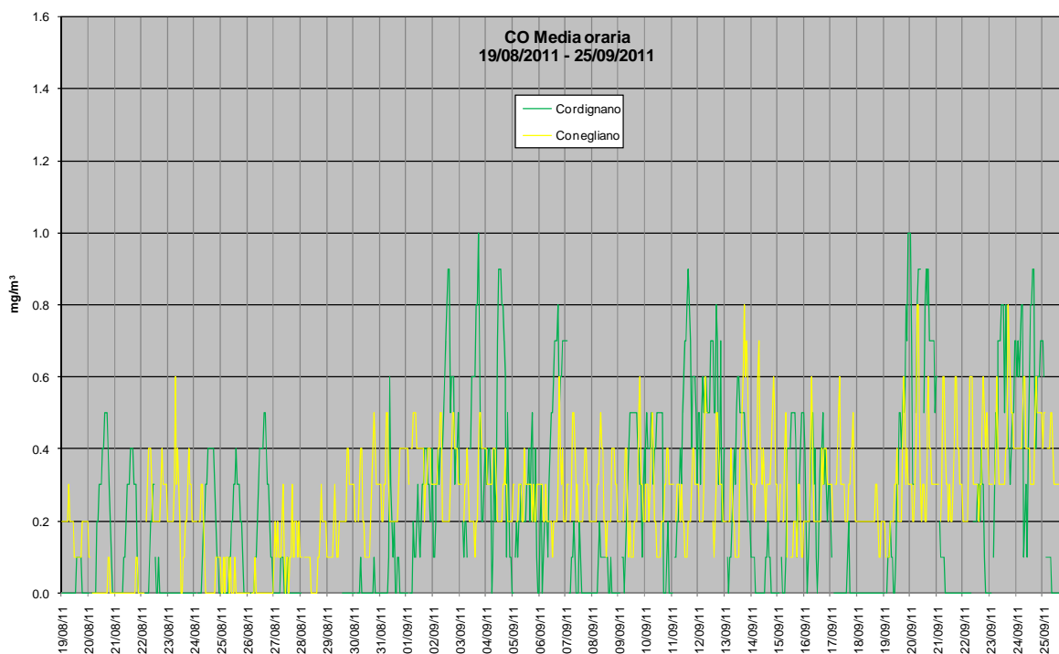
Grafico 2: Valori orari di CO rilevati presso la stazione fissa di Conegliano e la stazione rilocabile posizionata a Cordignano – campagna estiva.
