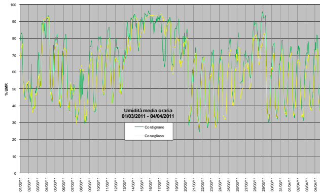
Grafico 19: Valori orari di umidità osservati presso la stazione rilocabile posizionata a Cordignano – campagna invernale
