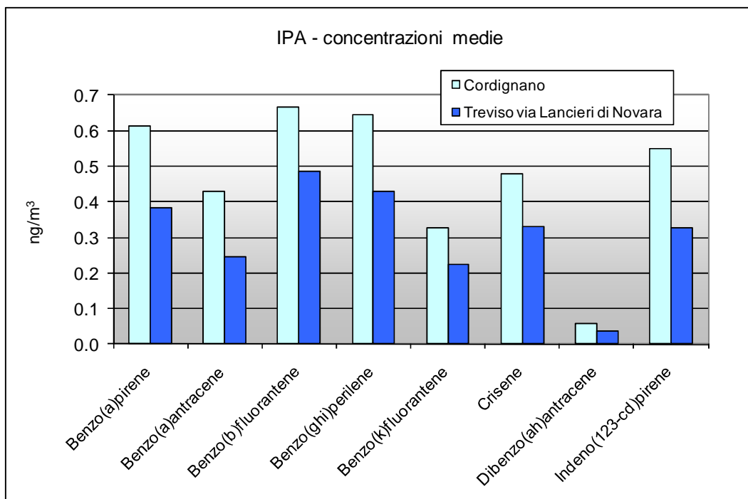
Grafico 21 Confronto tra i valori di IPA determinati su campioni di PM10 prelevati nel sito di monitoraggio e presso la stazione fissa di Treviso durante le campagne.
