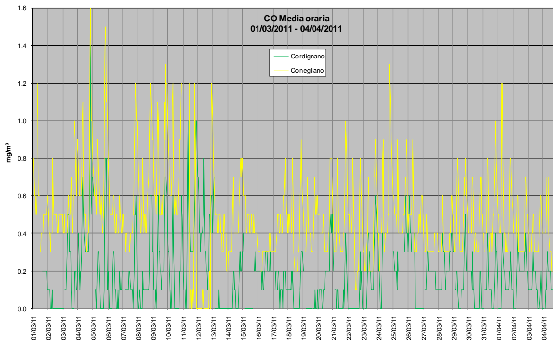
Grafico 1: Valori orari di CO rilevati presso la stazione fissa di Conegliano e la stazione rilocabile posizionata a Cordignano – campagna invernale.
