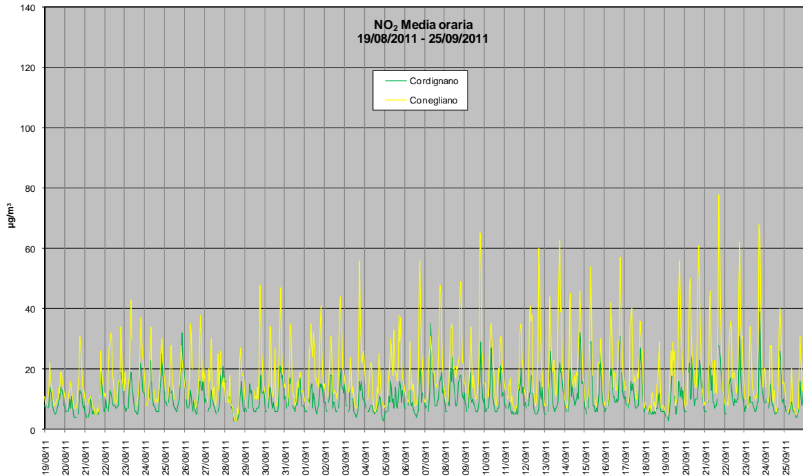
Grafico 4: Valori orari di NO 2 rilevati presso la stazione fissa di Conegliano e la stazione rilocabile posizionata a Cordignano – campagna estiva.
