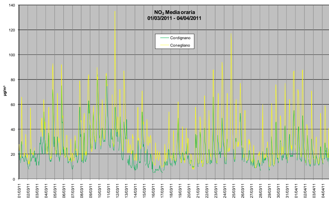
Grafico 3: Valori orari di \text{NO}_2 rilevati presso la stazione fissa di Conegliano e la stazione rilocabile posizionata a Cordignano – campagna invernale.
