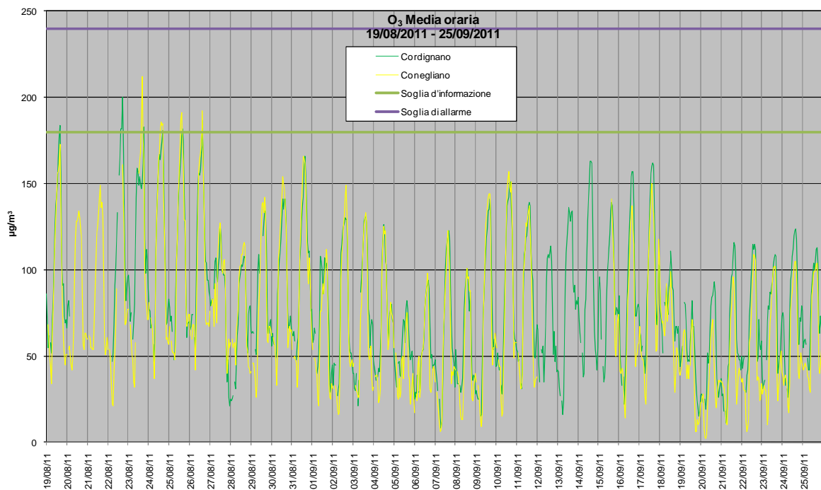
Grafico 6: Valori orari di O 3 rilevati presso la stazione fissa di Conegliano e la stazione rilocabile posizionata a Cordignano – campagna estiva.
