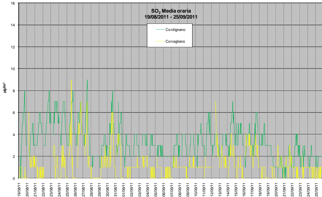
Grafico 8: Valori orari di SO 2 rilevati presso la stazione fissa di Conegliano e la stazione rilocabile posizionata a Cordignano – campagna estiva.
