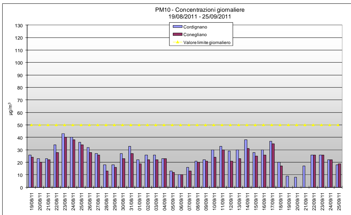
Grafico 11: Valori medi giornalieri di PM10 rilevati presso la stazione fissa di Conegliano e la stazione rilocabile posizionata a Cordignano – campagna estiva.
