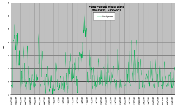
Grafico 13: Valori orari di velocità del vento osservati presso la stazione rilocabile posizionata a Cordignano – campagna invernale
