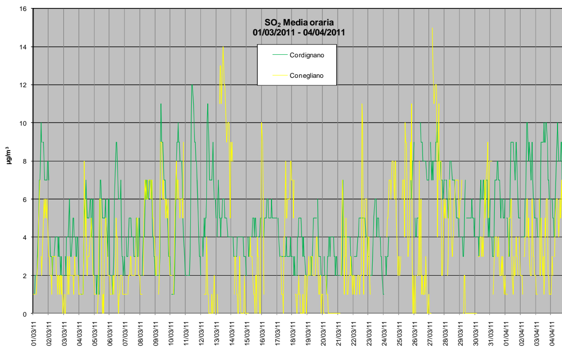
Grafico 7: Valori orari di SO 2 rilevati presso la stazione fissa di Conegliano e la stazione rilocabile posizionata a Cordignano – campagna invernale.
