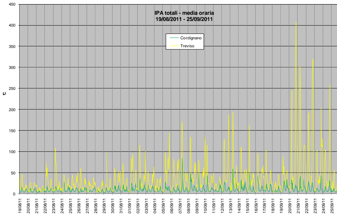
Grafico 9 Confronto tra le concentrazioni medie orarie di IPA totali in fase gassosa a Treviso e presso la stazione rilocabile posizionata a Cordignano – campagna estiva
