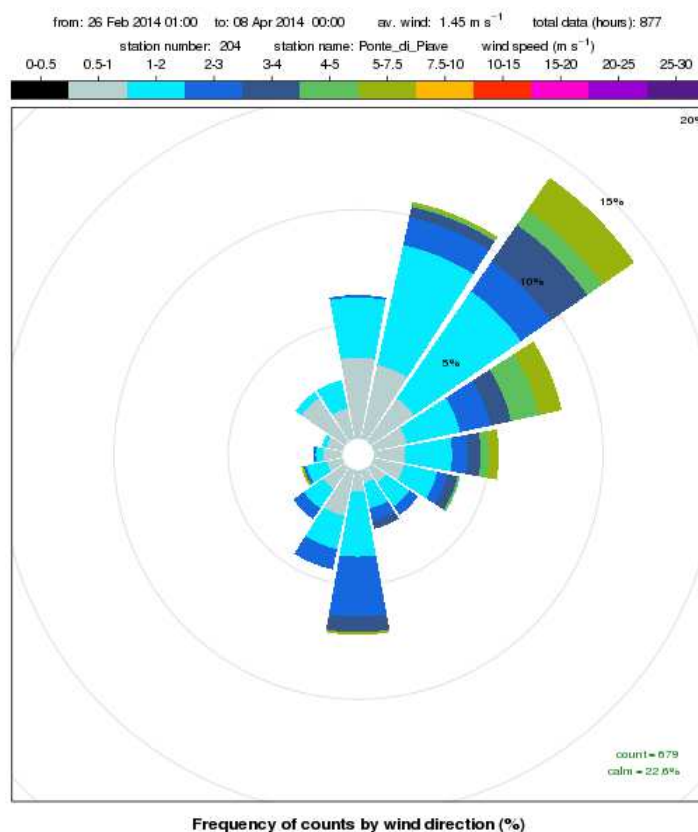
Figura 4. rosa dei venti a scansione oraria registrati presso la stazione meteorologica di Ponte di Piave nel periodo 26 febbraio – 7 aprile 2014
