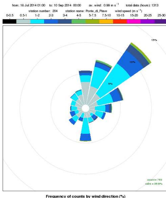
Figura 6. rosa dei venti a scansione oraria registrati presso la stazione meteorologica di Ponte di Piave nel periodo 16 luglio – 9 settembre 2014
