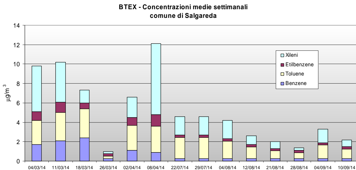
Grafico 2 - Valori settimanali di BTEX (benzene, toluene, etilbenzene e xilene) rilevati a Salgareda.
