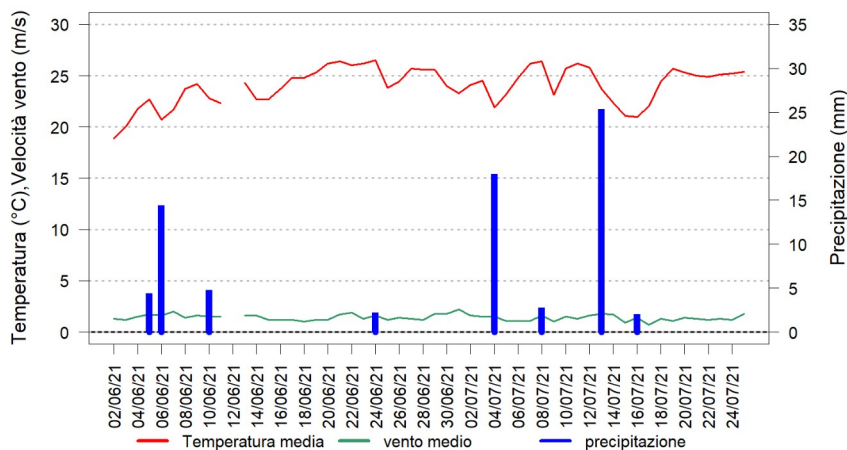
Andamento giornaliero dei parametri meteorologici a Fossalta di Portogruaro Periodo: 02/06/2021 - 25/07/2021
