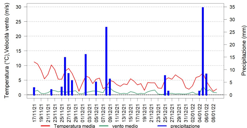
Andamento giornaliero dei parametri meteorologici a Fossalta di Portogruaro Periodo: 17/11/2021 - 09/01/2022
